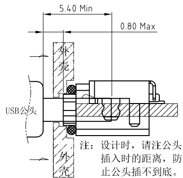
组装示意图
